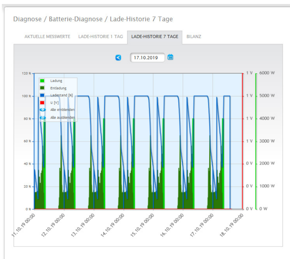
Abb.: Batterie-Diagnose - Lade Historie 7 Tage
