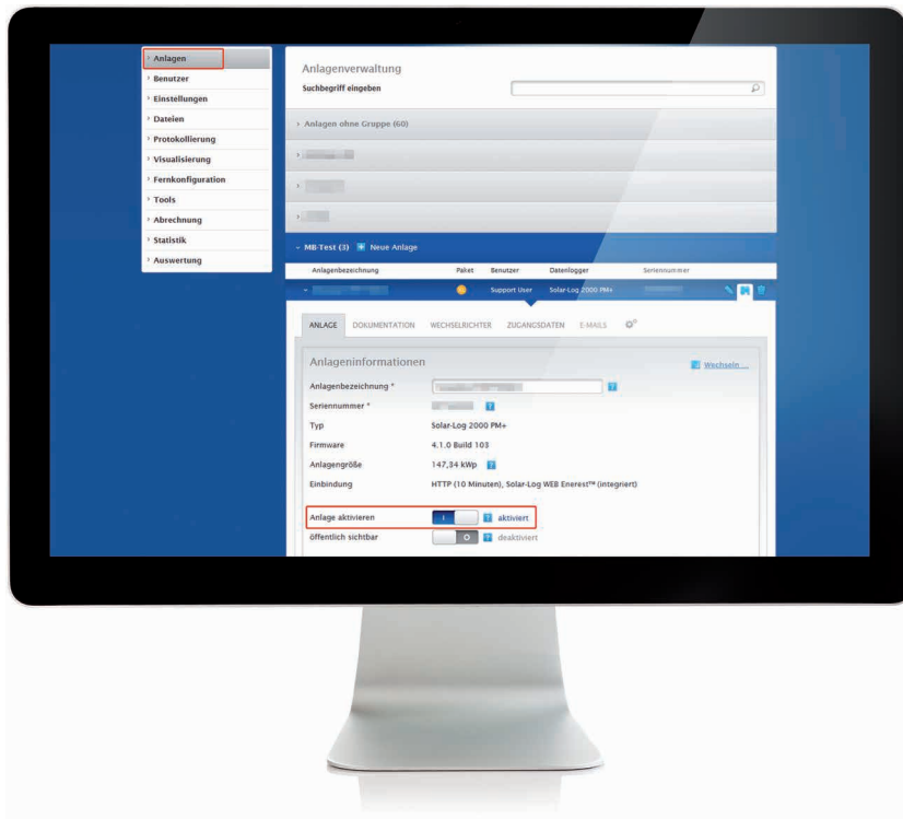
Anlage deaktivieren
