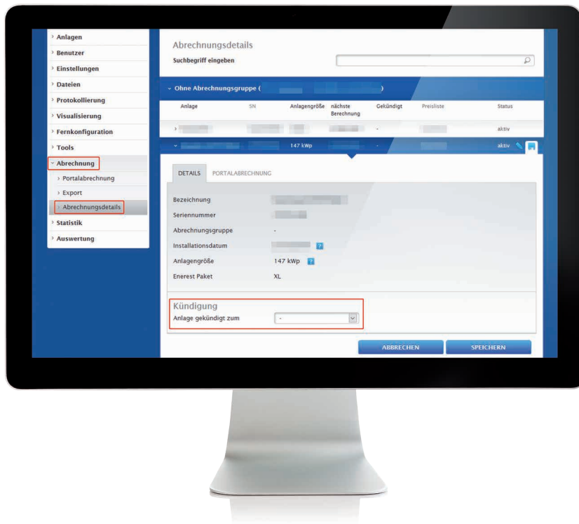
Kündigungsdatum setzen
