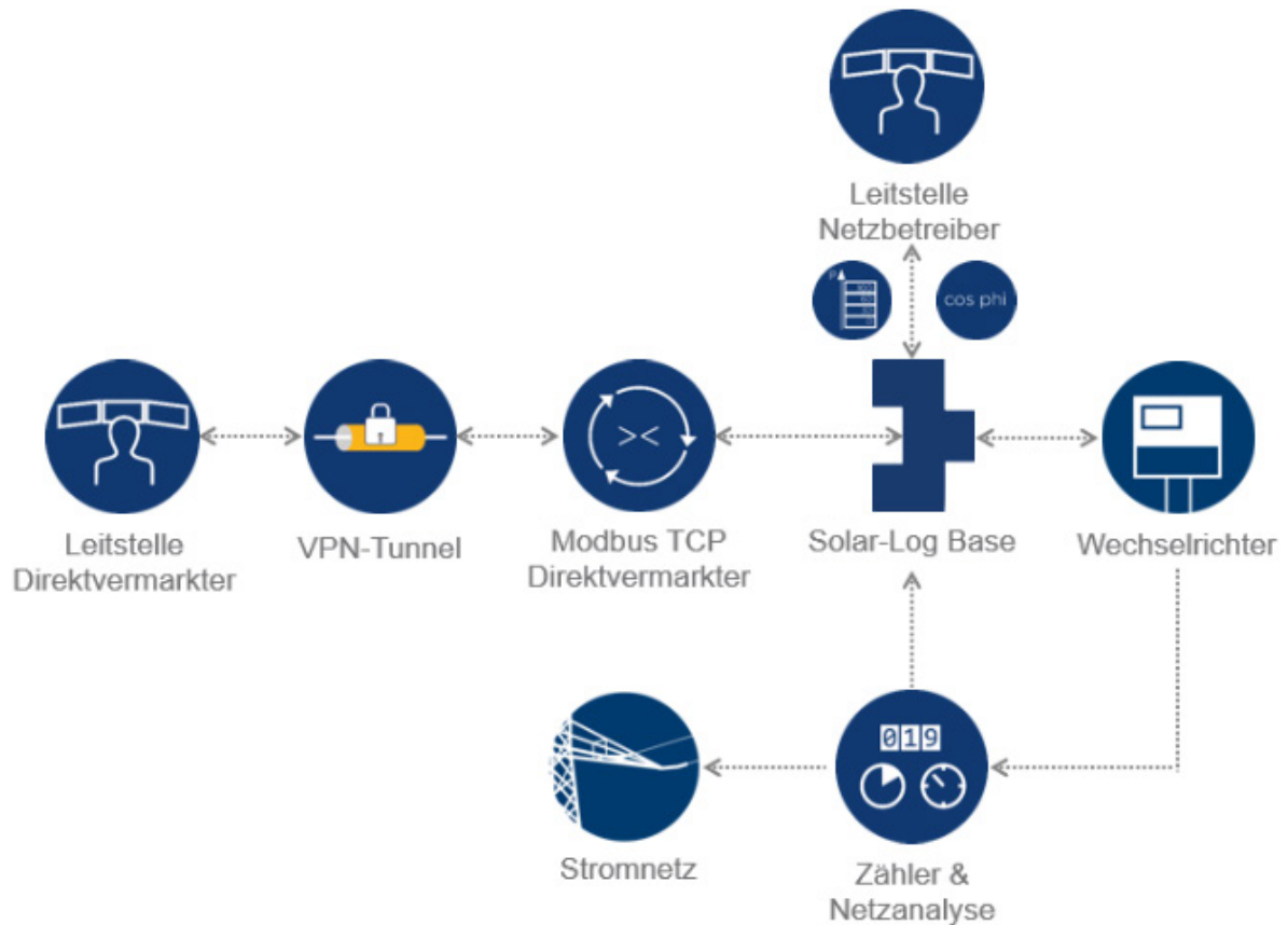
Schematischer Aufbau Direktvermarktung über Modbus TCP DPM
